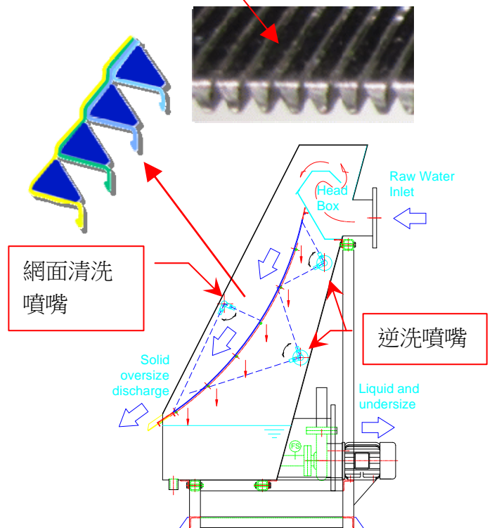
三角型篩網
